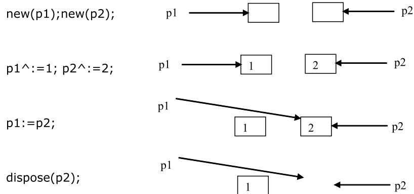
Рис. 8.2 – Создание и уничтожение динамических переменных
