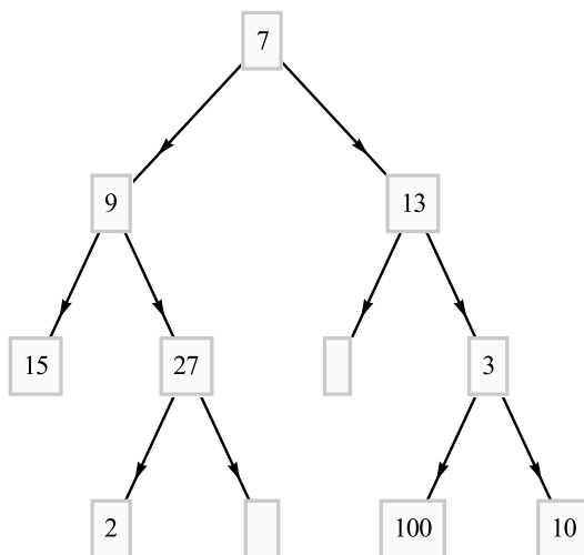
Рис. 8.9 – Пример бинарного дерева
