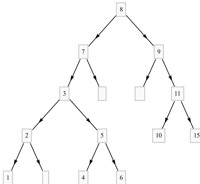
Рис. 8.10 – Упорядоченное бинарное дерево
