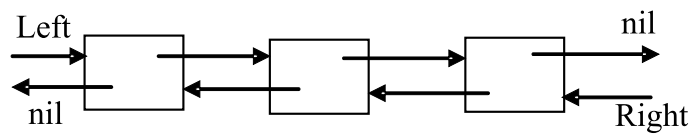
Рис. 8.6 – Список с двумя связями
