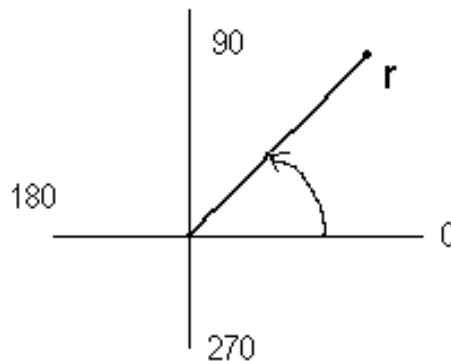
Рис. 9.3 – Полярная система координат
